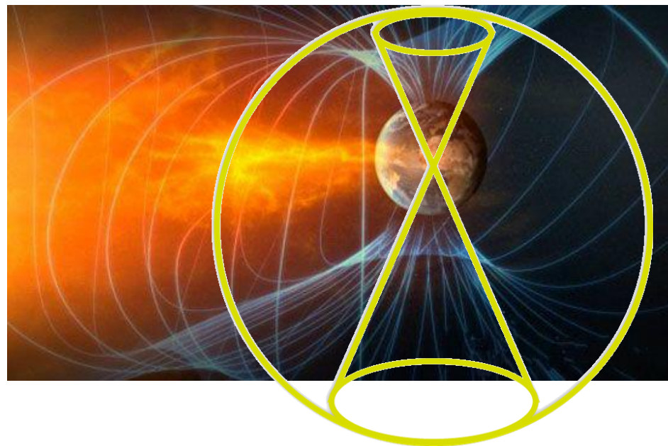
地球磁力线与磁场模型图
